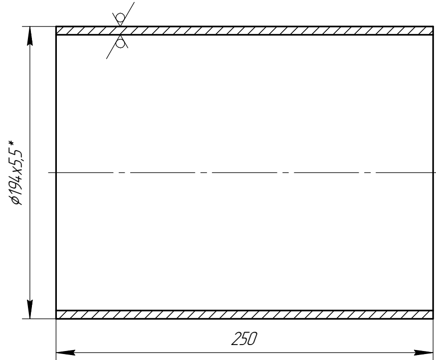
Дет. поз. 4
