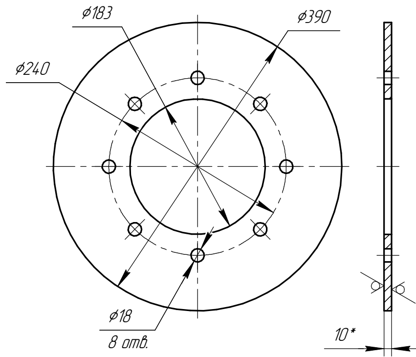
Дет. поз. 2 (1:5)
