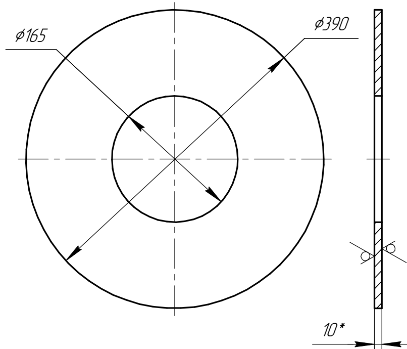
Дет. поз. 1 (1:5)
