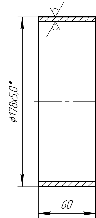
Дет. поз. 5
