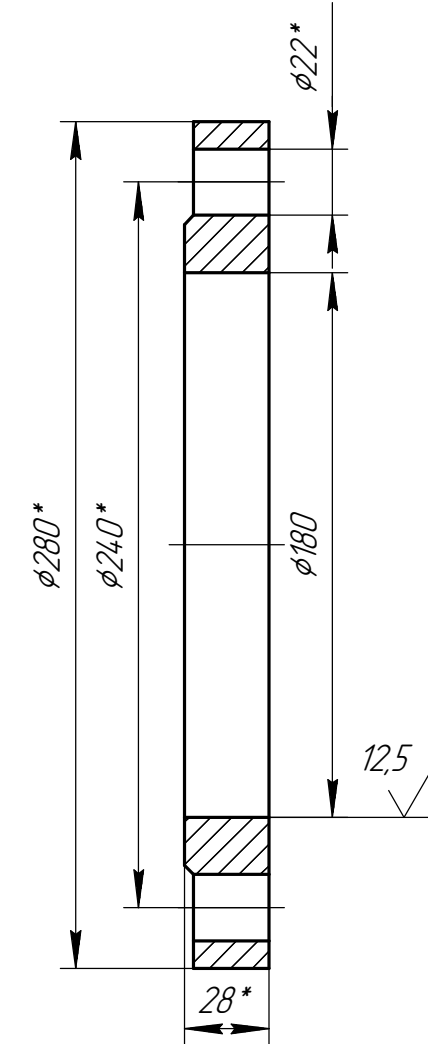
Дет. поз. 6
