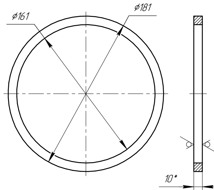
Дет. поз. 3
